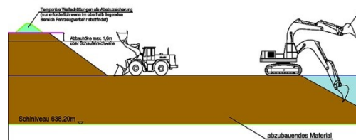
Schema Abbauvorgang M 1:250
